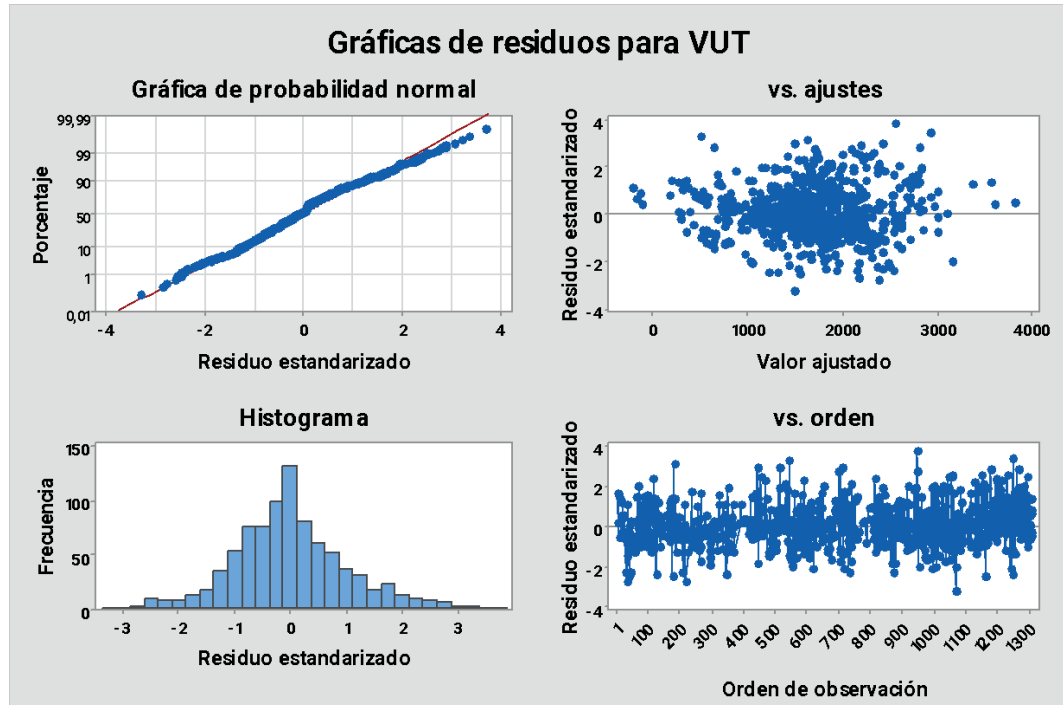
Figura 2. Cumplimiento de los supuestos del ARM. Estadístico de Durbin-Watson = 1.79426
